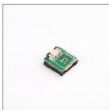
Zino00-07 Gyro Module
